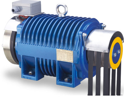
SMT Serisi Dişlisiz Tahrik Motoru ve Tahrik Kasnağı SMT Series Traction Motor and Traction Sheave
